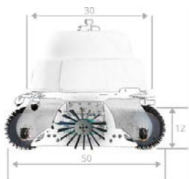
Dimensiones/Dimensions
